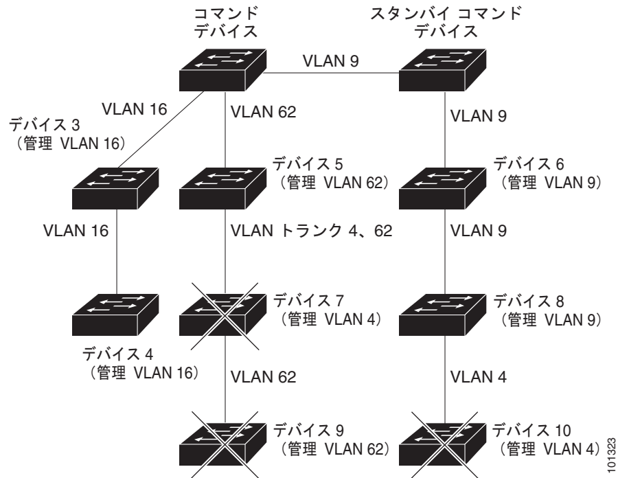
図 5-4 レイヤ 3 クラスター コマンド スイッチを使用して異なる管理 VLAN から検出
