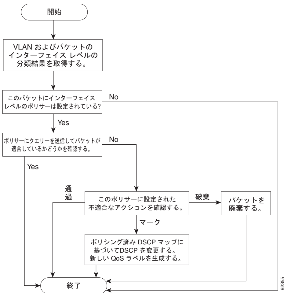
図 35-5 SVI のポリシングおよびマーキング フローチャート
