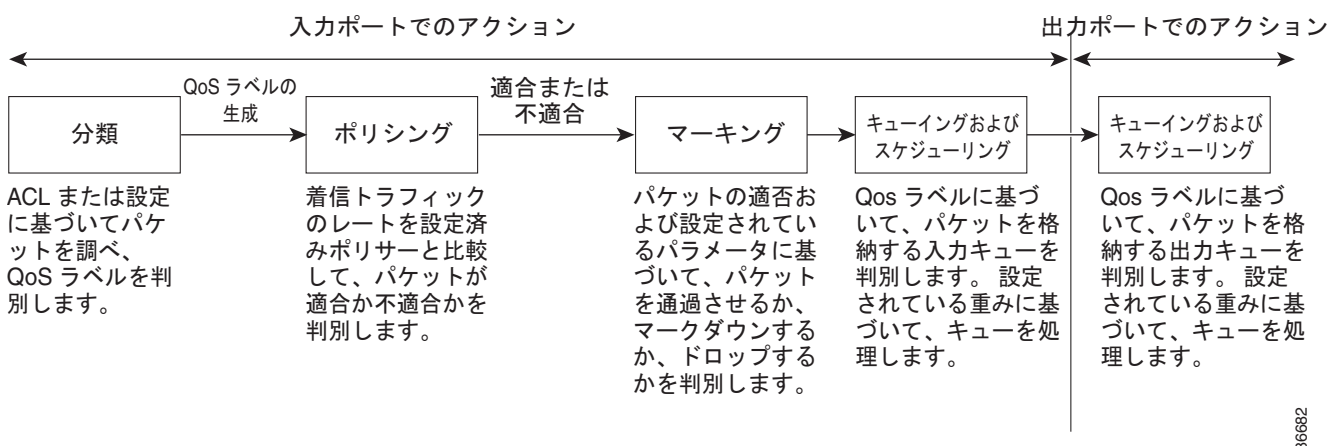
図 35-2 QoS の基本モデル
