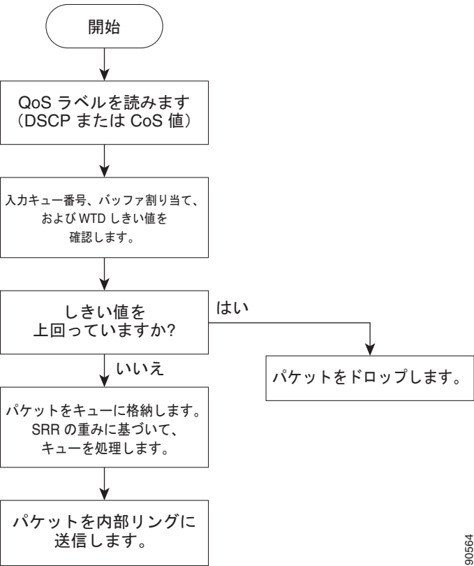
図 35-8 入力ポートのキューイングおよびスケジューリング フローチャート
