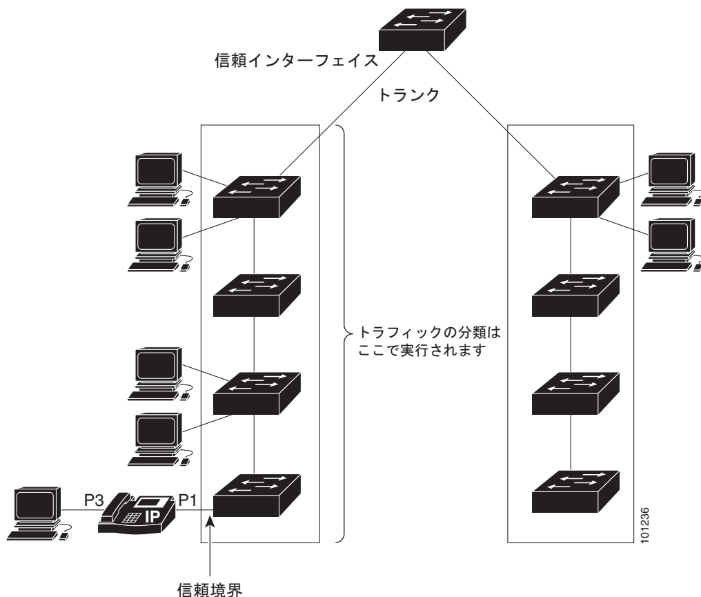
図 35-12 QoS ドメイン内のポートの信頼状態
