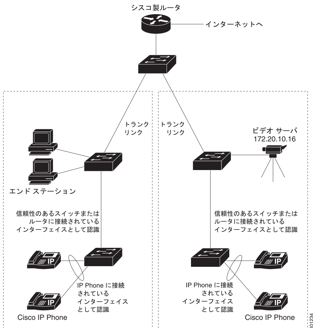
図 35-11 ネットワークでの自動 QoS の設定例
