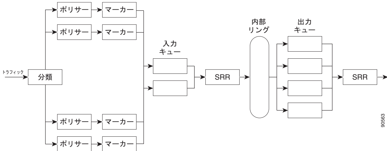
図 35-6 入力および出力キューの位置
