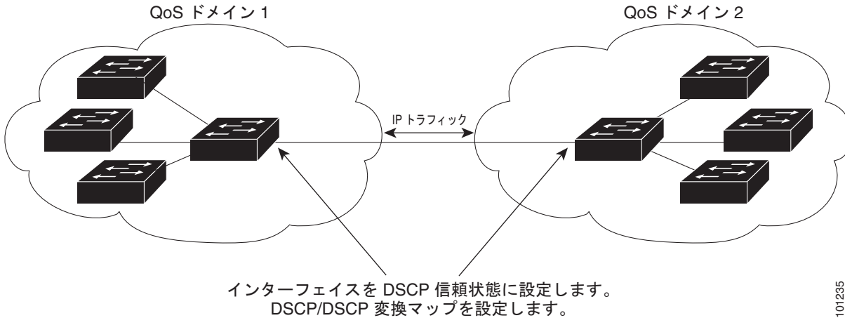
図 35-13 別の QoS ドメインとの境界ポートの DSCP 信頼状態
