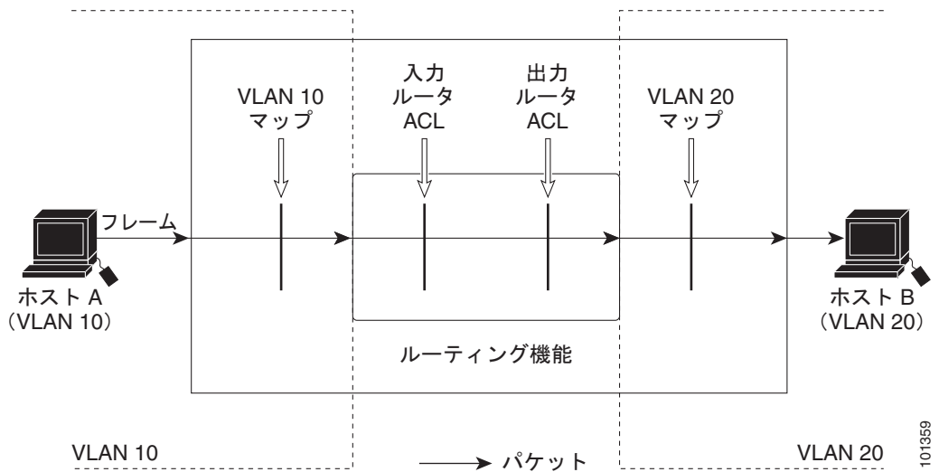
図 34-8 ルーテッド packets への ACL の適用
