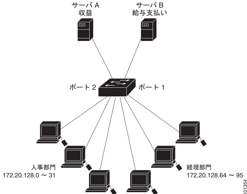
図 34-3 ルータ ACL によるトラフィックの制御
