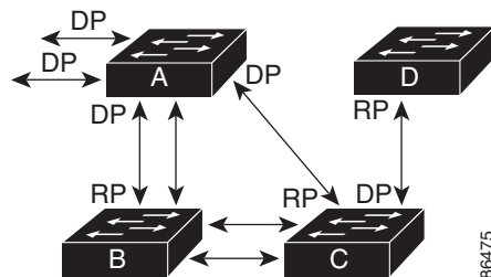
図 18-2 スパンニング ツリー トポロジ
