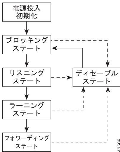
図 18-1 スパンニング ツリー インターフェイス ステート
