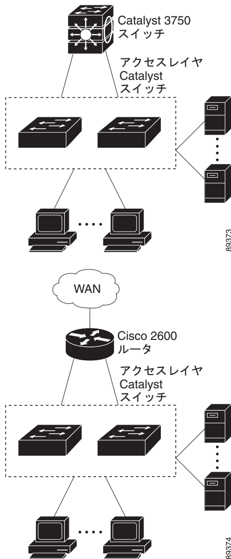
図 1-1 高性能なワークグループ (GTTD)
