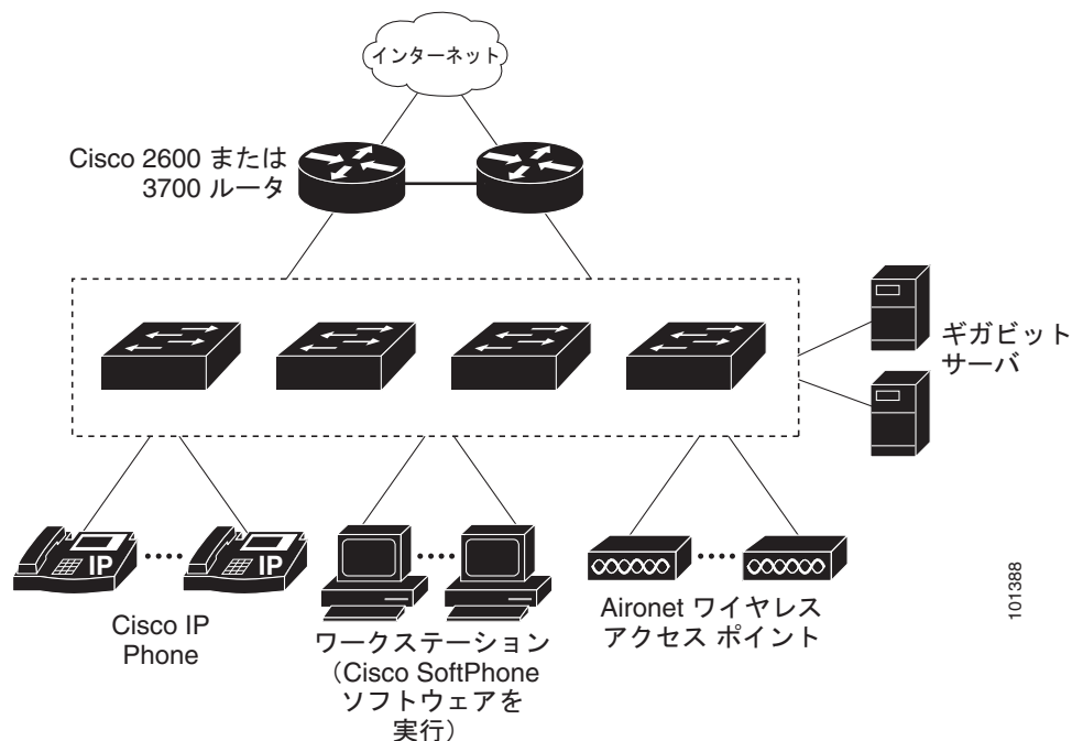
図 1-3 コラプスト バックボーン構成の Catalyst 3560 スイッチ
