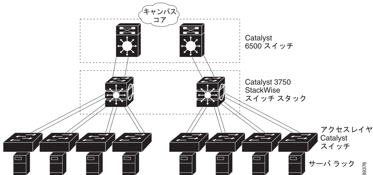
図 1-2 サーバ集約
