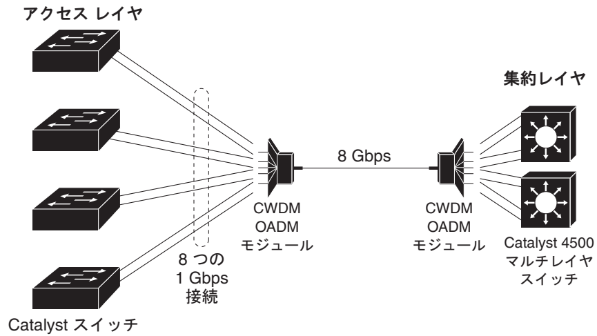
図 1-5 長距離広帯域トランスポートの構成
