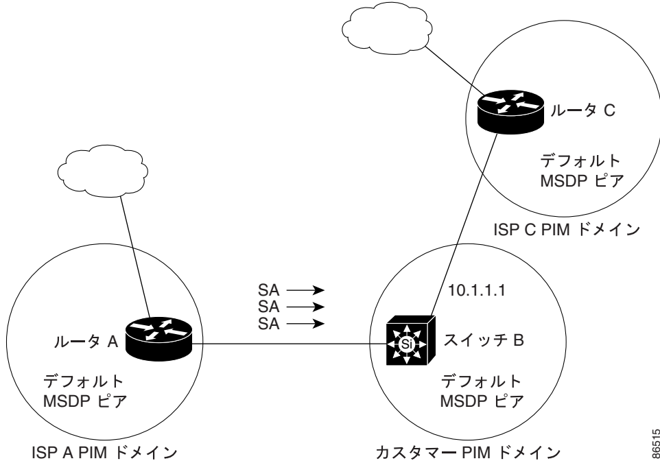
図 42-2 デフォルトの MSDP ピア ネットワーク
