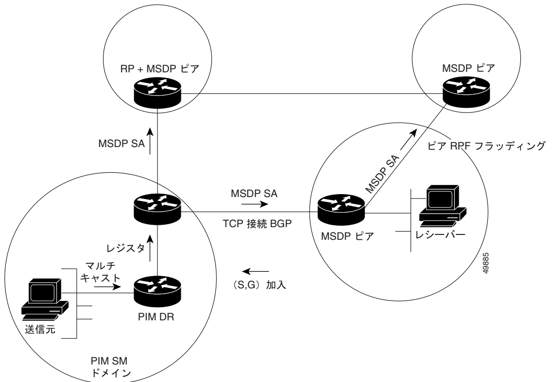
図 42-1 RP ピア間で動作する MSDP
