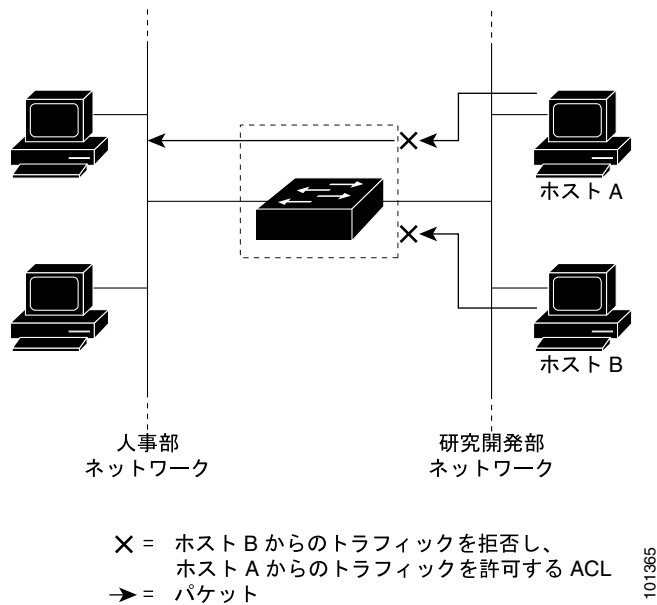
図 32-1 ACL を使用したネットワーク トラフィックの制御
