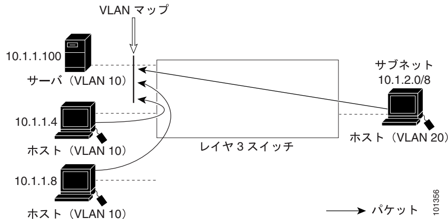
図 32-5 他の VLAN 上のサーバへのアクセス拒否
