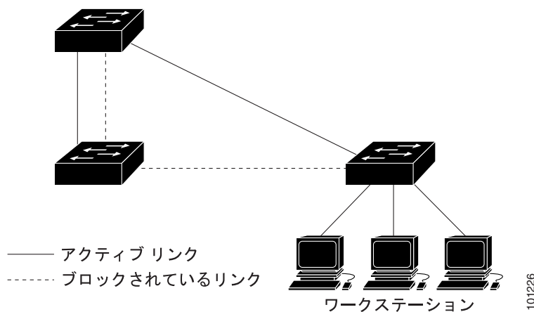
図 17-3 スパニング ツリーおよび冗長接続
