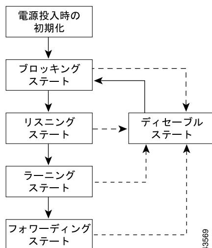
図 17-1 スパニング ツリー インターフェイス ステート
