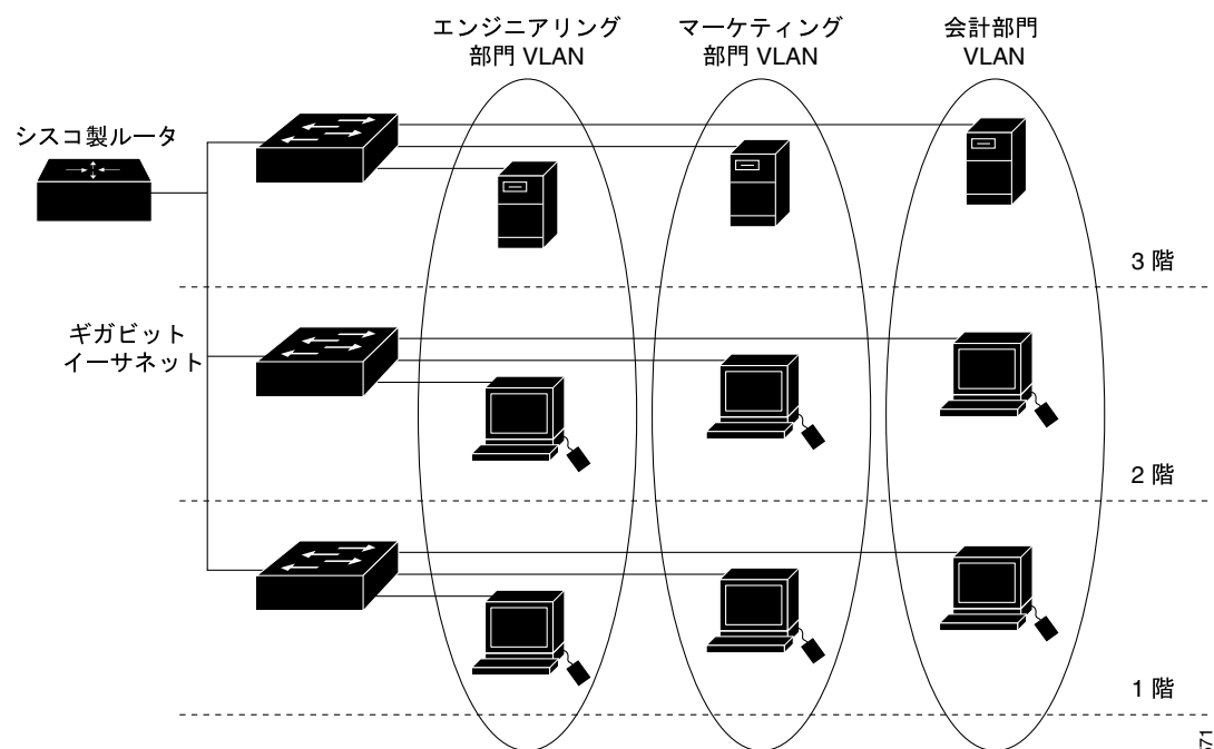
図 12-1 論理的に定義されたネットワークとしての VLAN
