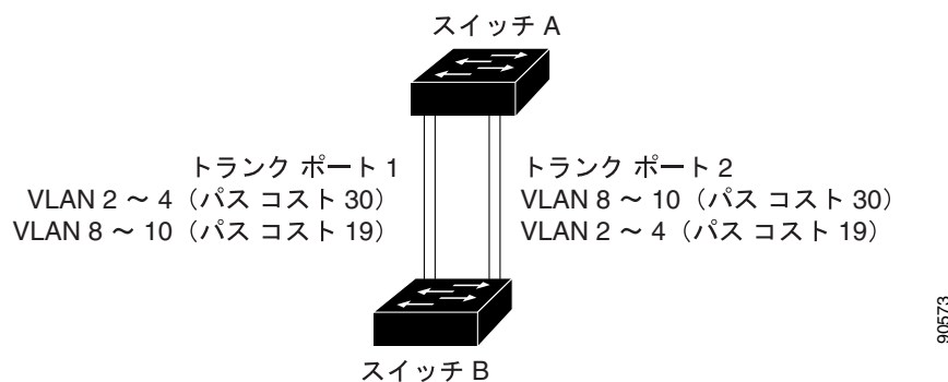
図 12-4 パス コストによってトラフィックが分散されるロード シェアリング トランク
