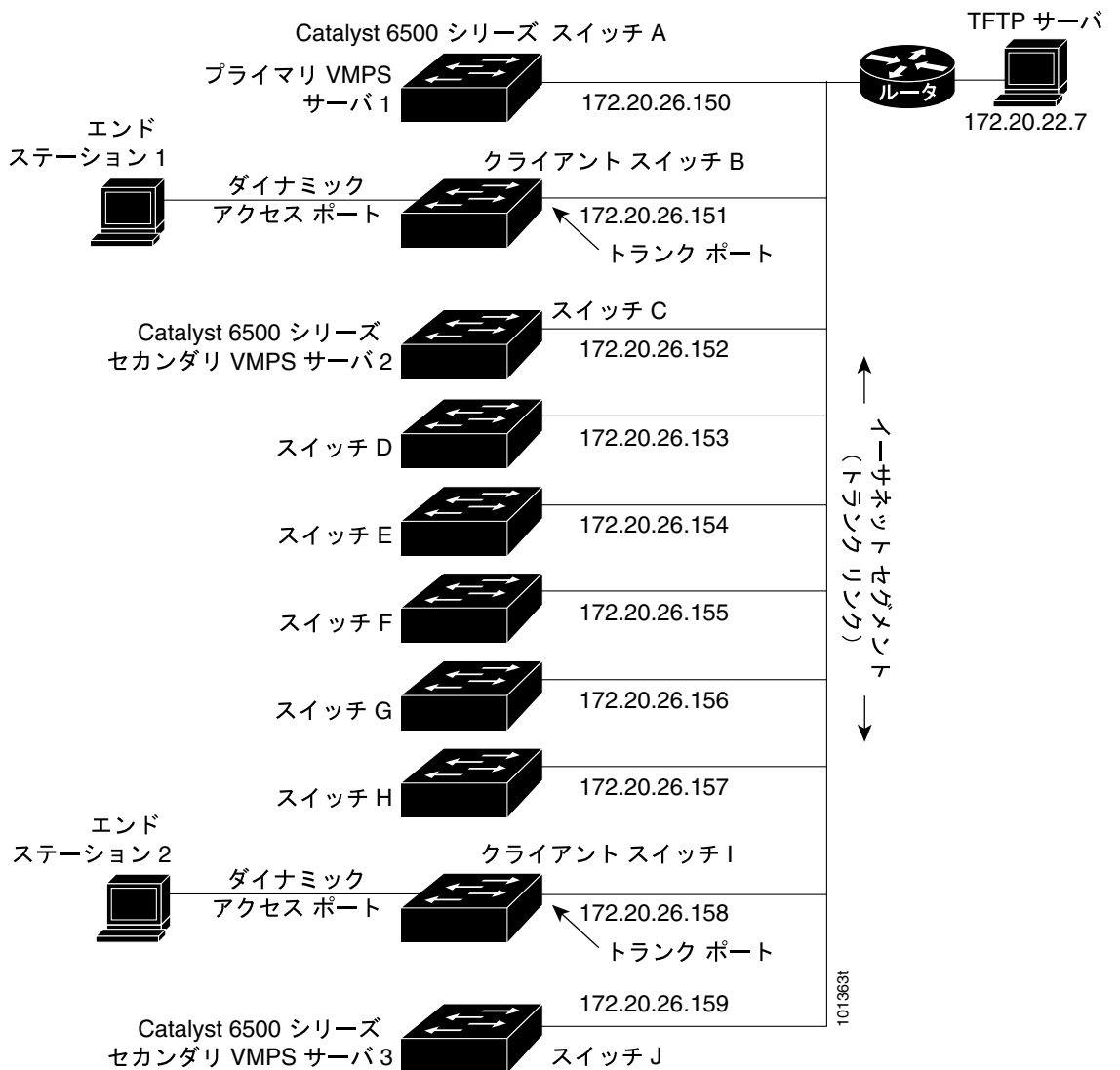
図 12-5 ダイナミック ポート VLAN メンバシップの構成例
