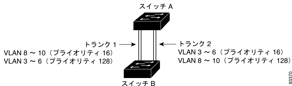
図 12-3 STP ポート プライオリティによるロード シェアリング
