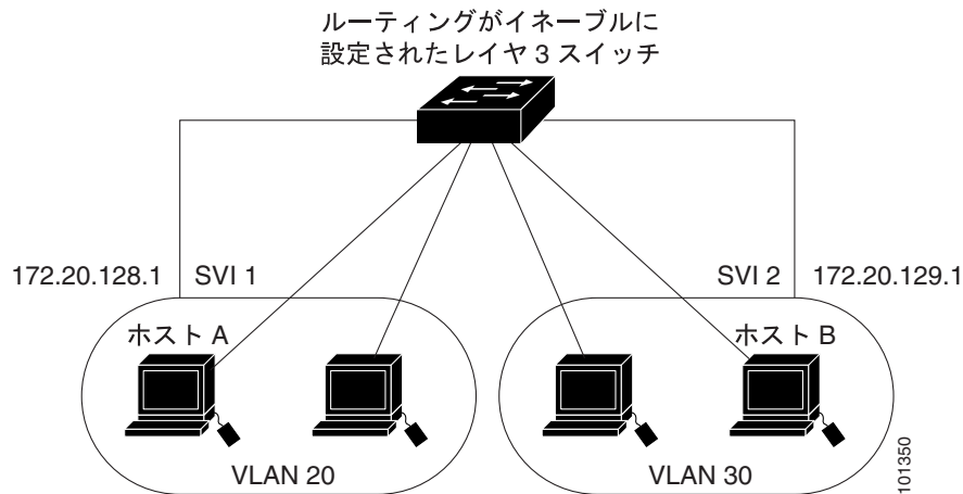
図 10-1 Catalyst 3560 スイッチによる VLAN の接続
