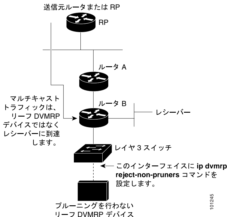
図 39-7 ルータが非ブルーニング DVMRP ネイバを拒否する例
