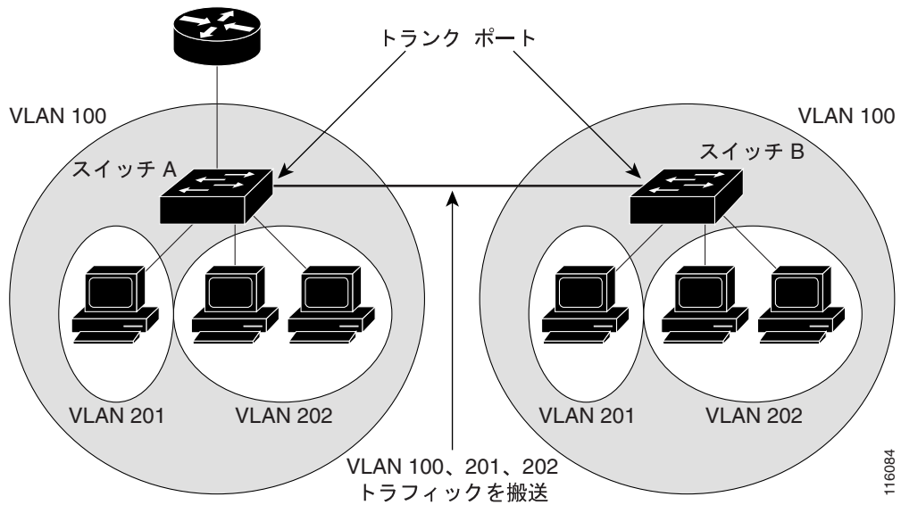
図 14-2 複数のスイッチにまたがるプライベート VLAN
