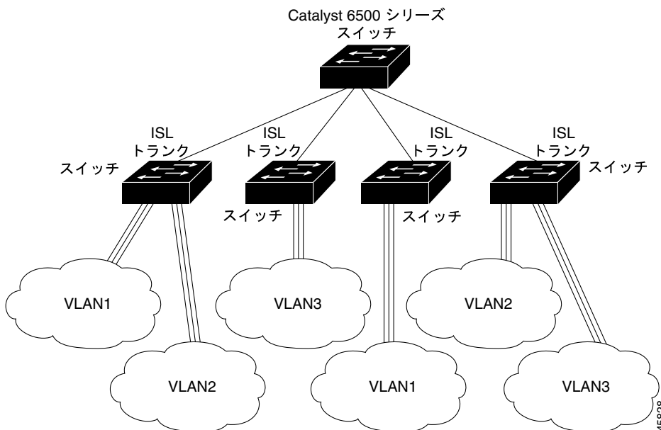
図 12-2 ISL トランキング環境のスイッチ
