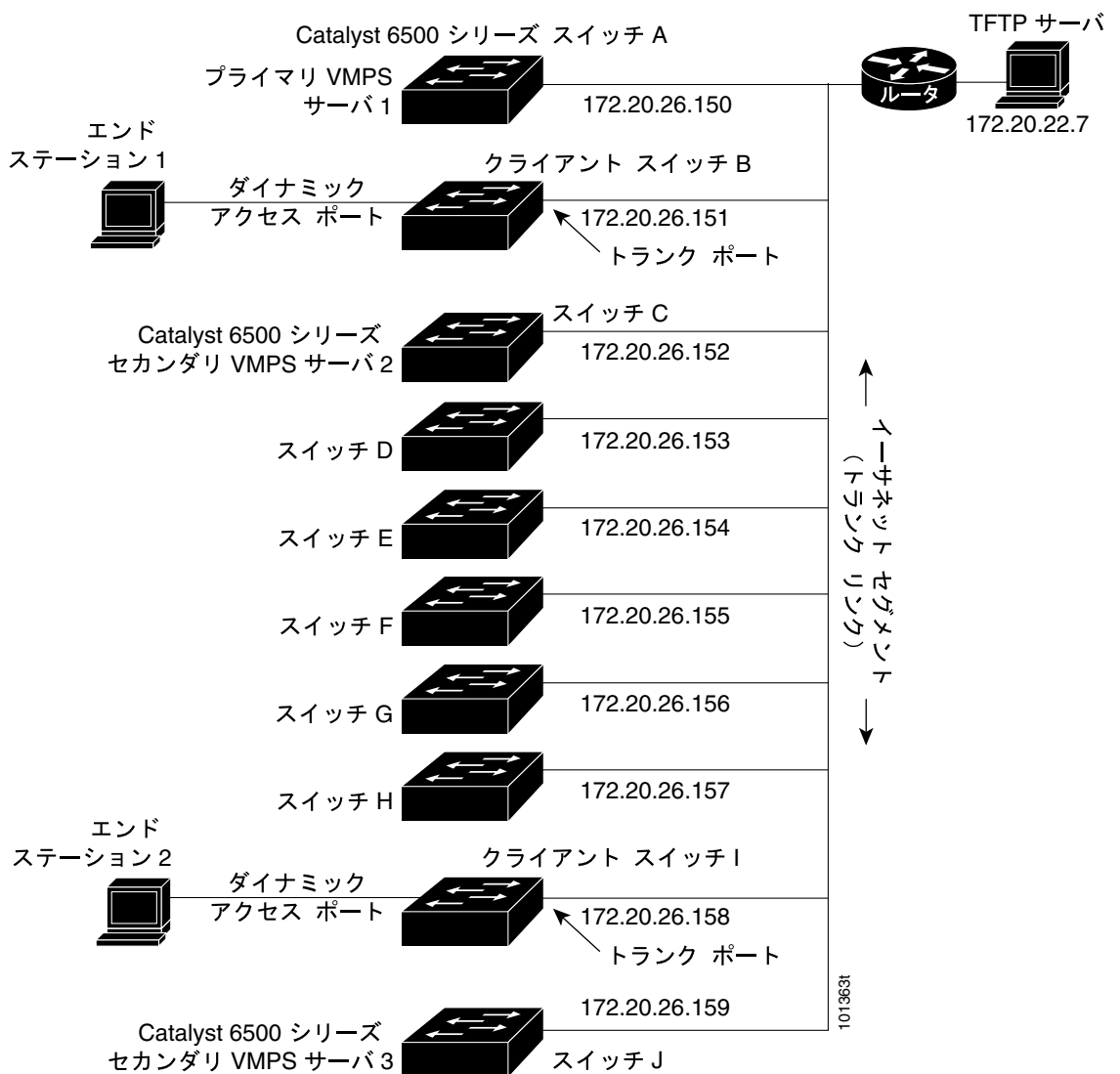
図 12-5 ダイナミック ポート VLAN メンバーシップの構成例
