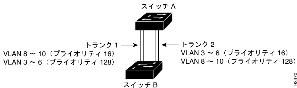
図 12-3 STP ポートプライオリティによる負荷分散
