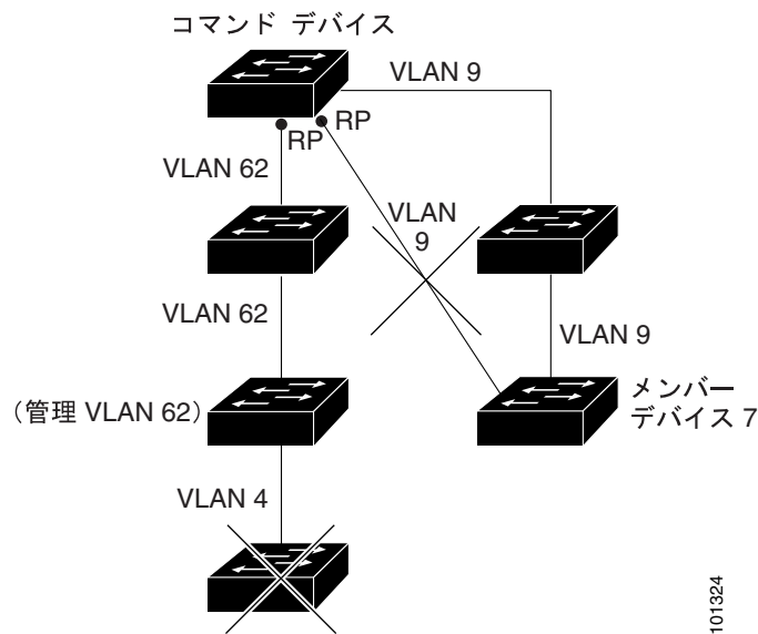
図 5-5 RP による検出
