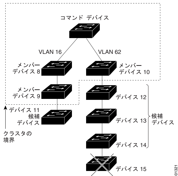
図 5-1 CDP ホップを使用しての検出
