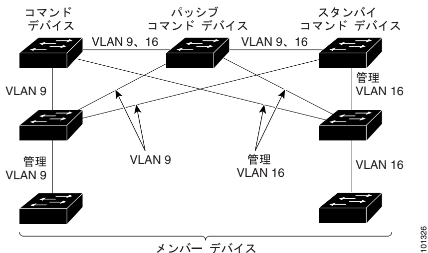
図 5-7 スタンバイグループメンバーとクラスタ メンバー間の VLAN 接続
