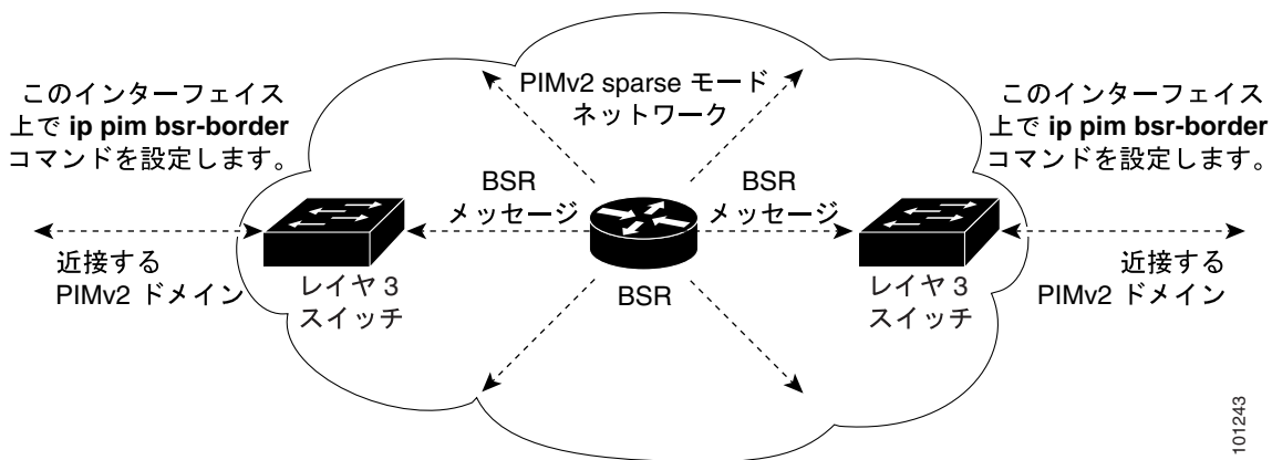
図 39-3 PIMv2 BSR メッセージの抑制
