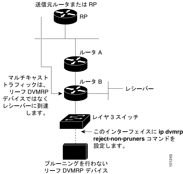
図 39-7 ルータが非プルーニング DVMRP ネイバを拒否する例
