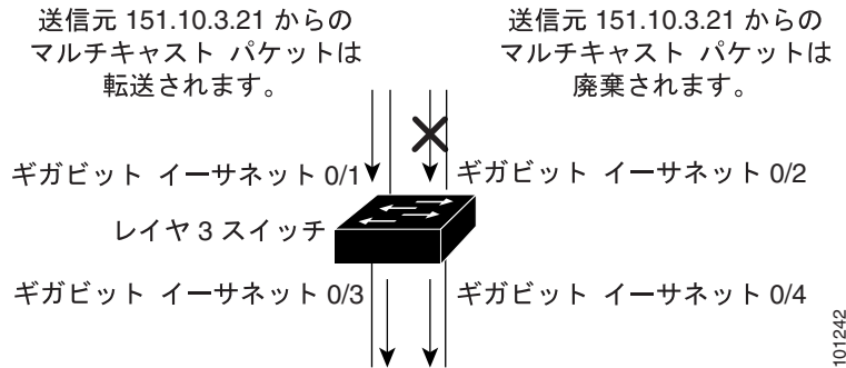
図 39-2 RPF チェック
