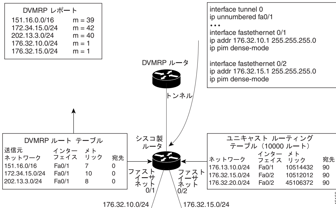
図 39-8 接続されたユニキャスト ルートにのみアドバタイズ (デフォルト) する例
