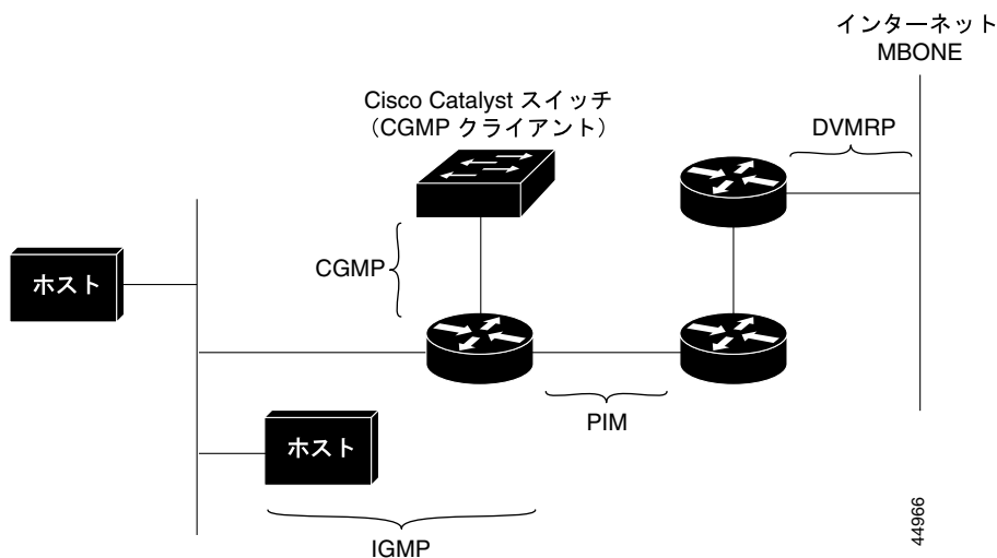
図 39-1 IP マルチキャストルーティング プロトコル
