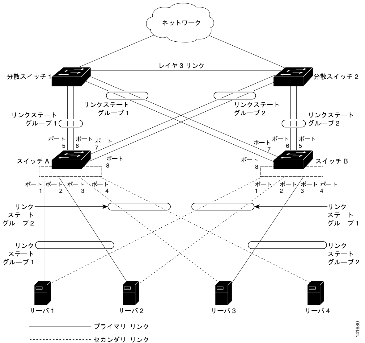
図 33-4 一般的なリンクステート追跡の設定
