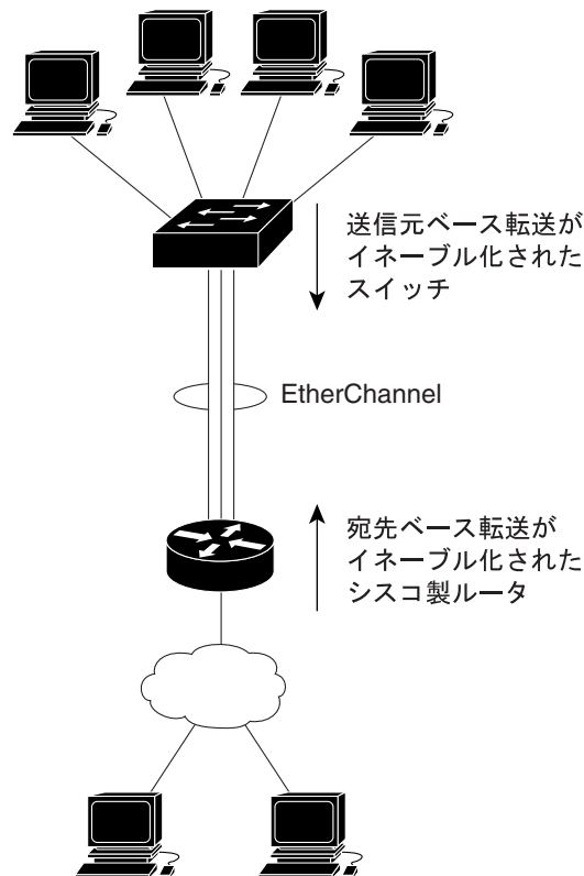
図 33-3 負荷の分散および転送方式
