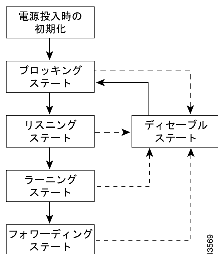
図 17-1 スパンニングツリー インターフェイス ステート
