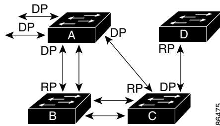
図 17-2 スパニングツリー トポロジー
