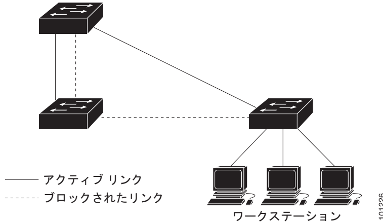
図 17-4 スパンニングツリーおよび冗長接続
