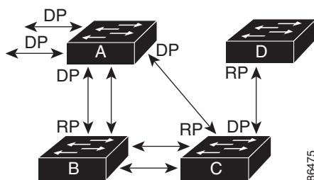
図 17-3 スパニングツリー トポロジー
