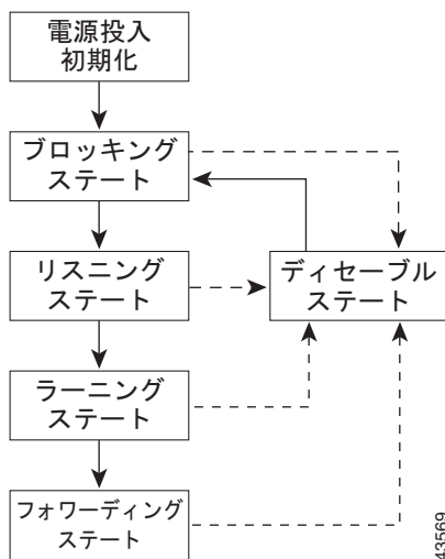
図 17-2 スパニングツリー インターフェイス ステート
