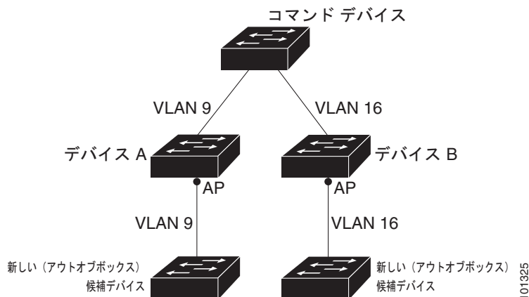
図 5-5 新しくインストールしたスイッチの検出
