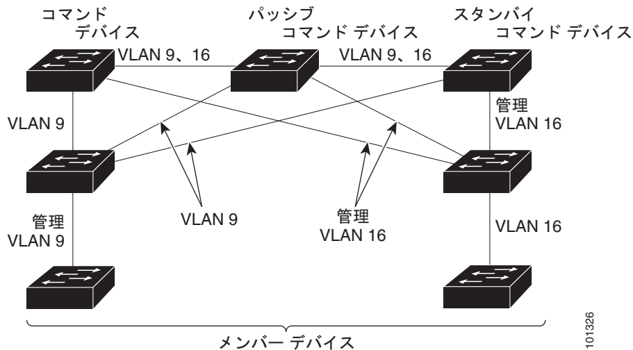
図 5-6 スタンバイグループメンバーとクラスタメンバー間の VLAN 接続
