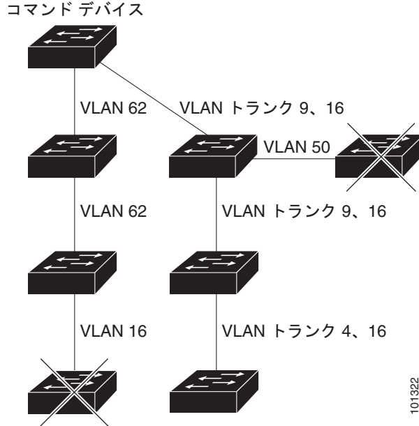
図 5-3 異なる VLAN からの検出
