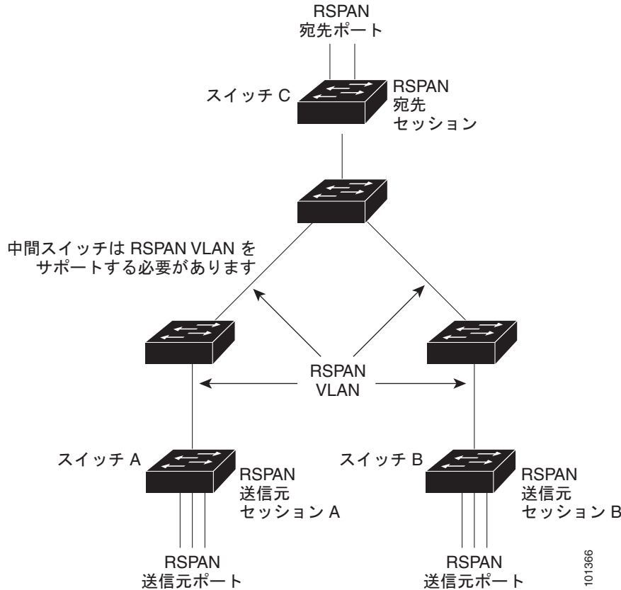
図 26-3 RSPAN の設定例
