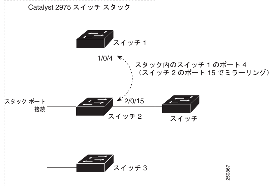
図 26-2 スイッチ スタックでのローカル SPAN の設定例
