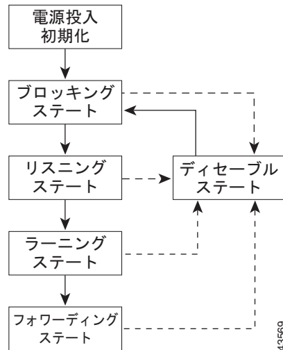
図 16-2 スパンニング ツリー インターフェイス ステート
