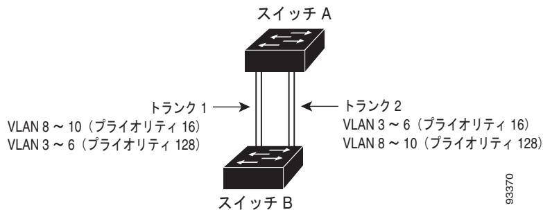
図 12-2 STP ポートプライオリティによる負荷分散
