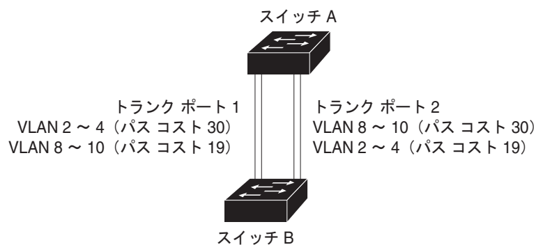
図 12-3 パス コストによってトラフィックが分散される負荷分散トランク
