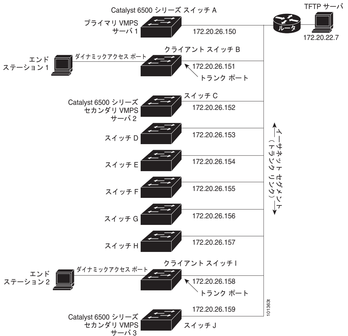
図 12-4 ダイナミック ポート VLAN メンバシップの構成例
