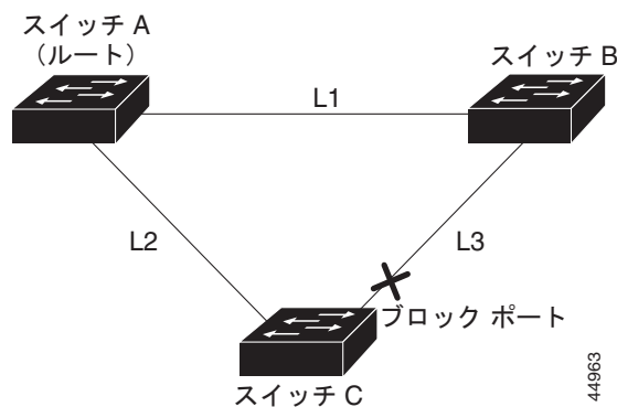
図 17-5 間接リンク障害発生前の BackboneFast の例
