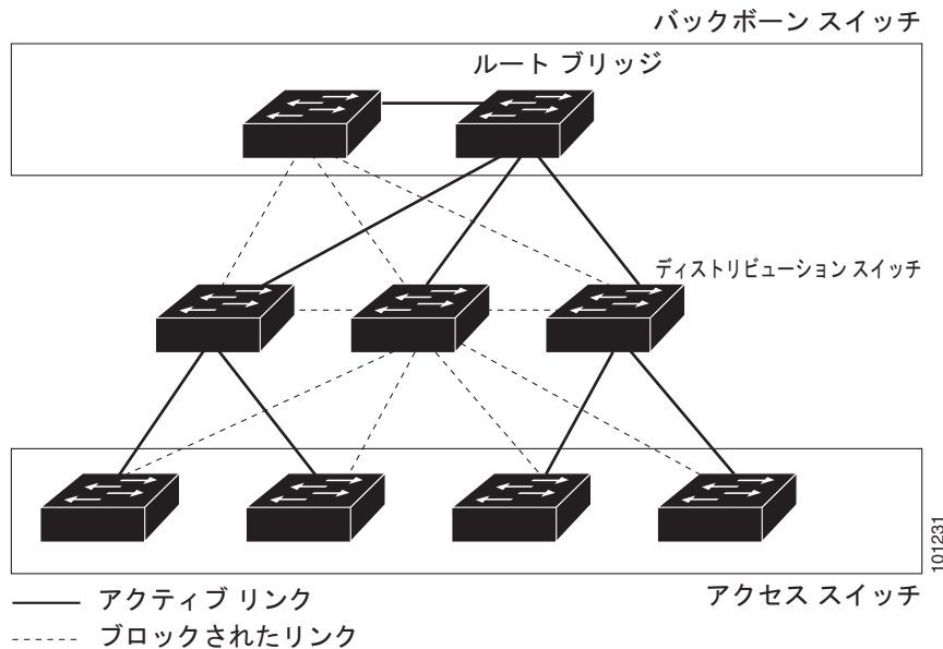
図 17-2 階層型ネットワークのスイッチ
