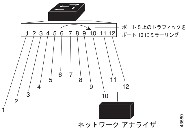
図 26-1 単一スイッチでのローカル SPAN の設定例
