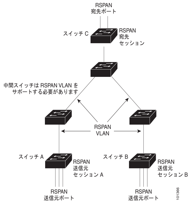
図 26-2 RSPAN の設定例
