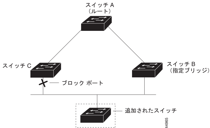
図 17-7 メディア共有型トポロジにおけるスイッチの追加
