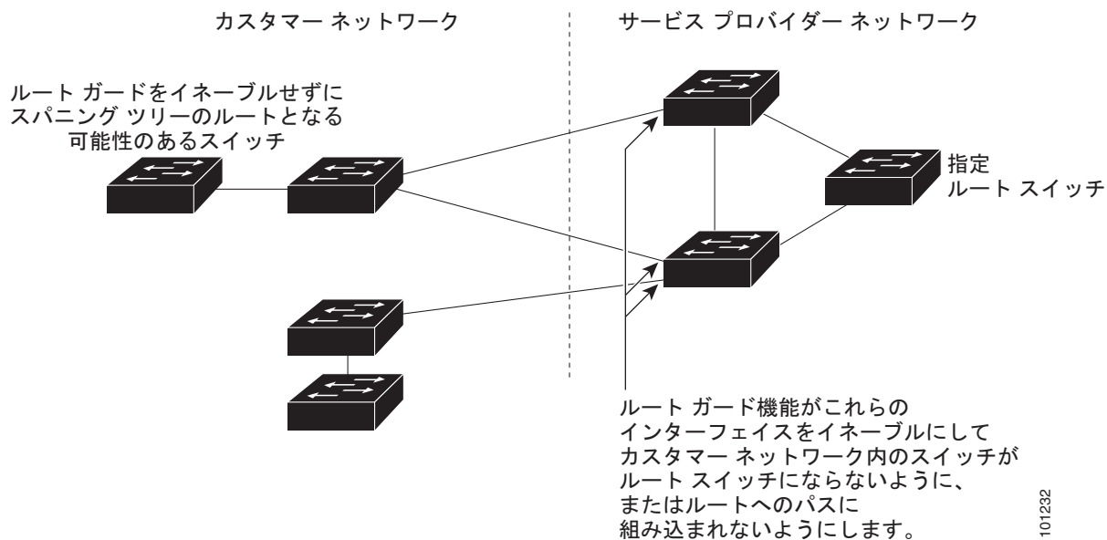
図 17-8 サービス プロバイダー ネットワークのルート ガード
