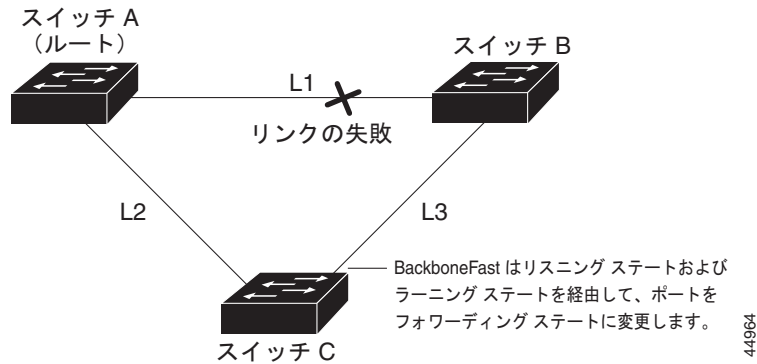
図 17-6 間接リンク障害発生後の BackboneFast の例
