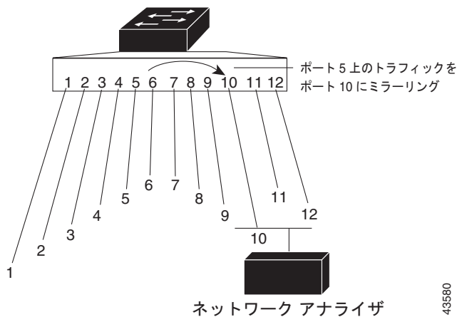
図 25-1 単一スイッチでのローカル SPAN の設定例
