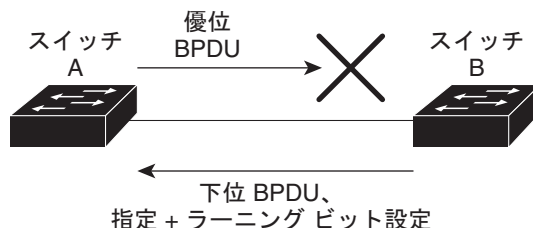
図 16-3 単一方向リンクの失敗の検出
