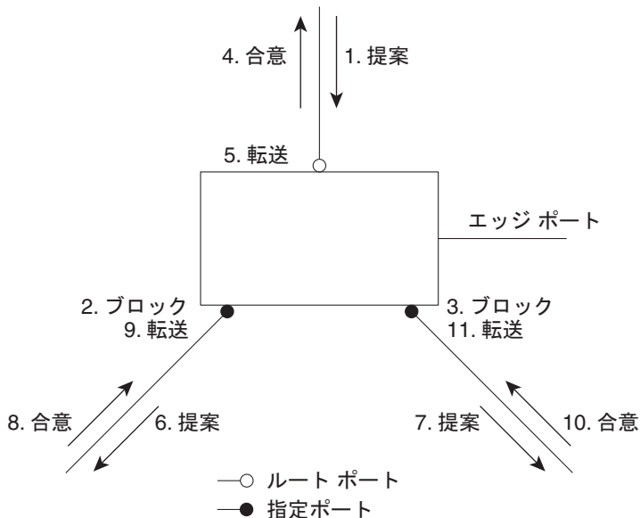
図 16-5 高速コンバージェンス中の一連のイベント
