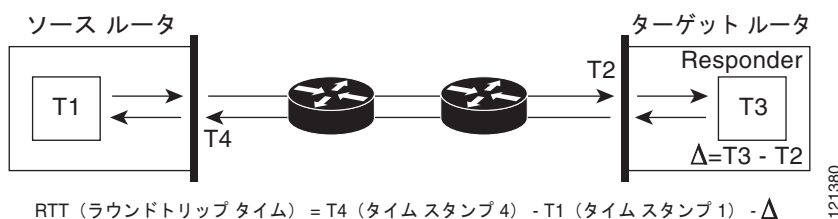
図 30-2 Cisco IOS IP SLA responder タイム スタンプ
