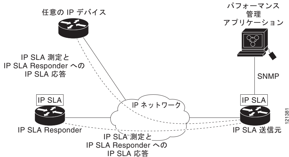
図 30-1 Cisco IOS IP SLA 動作
