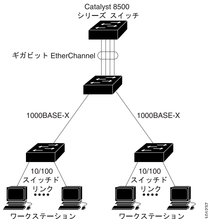
図 28-1 一般的な EtherChannel 構成
