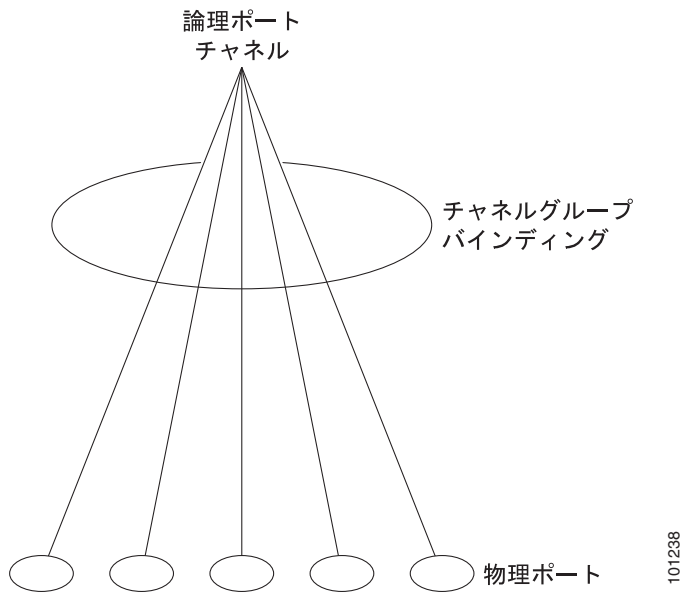
図 28-2 物理ポート、論理ポートチャンネル、およびチャンネルグループの関係
