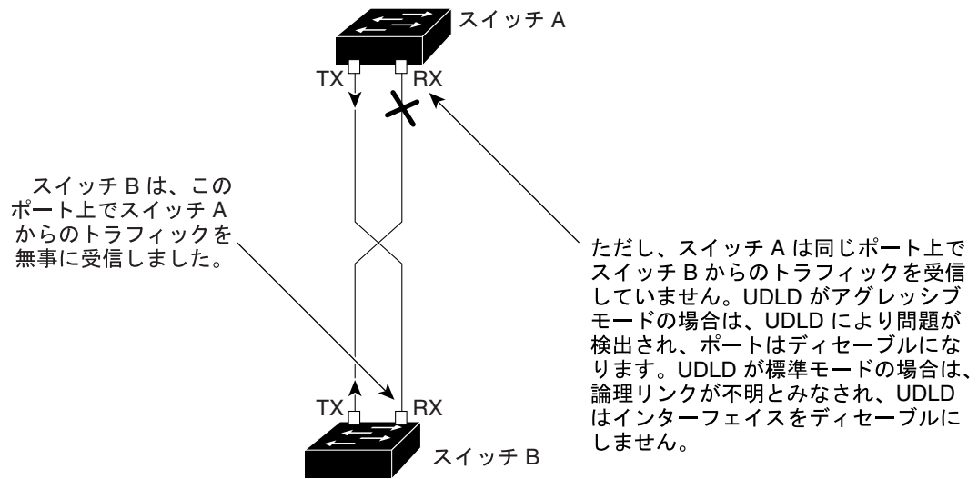
図 22-1 UDLD による単一方向リンクの検出
