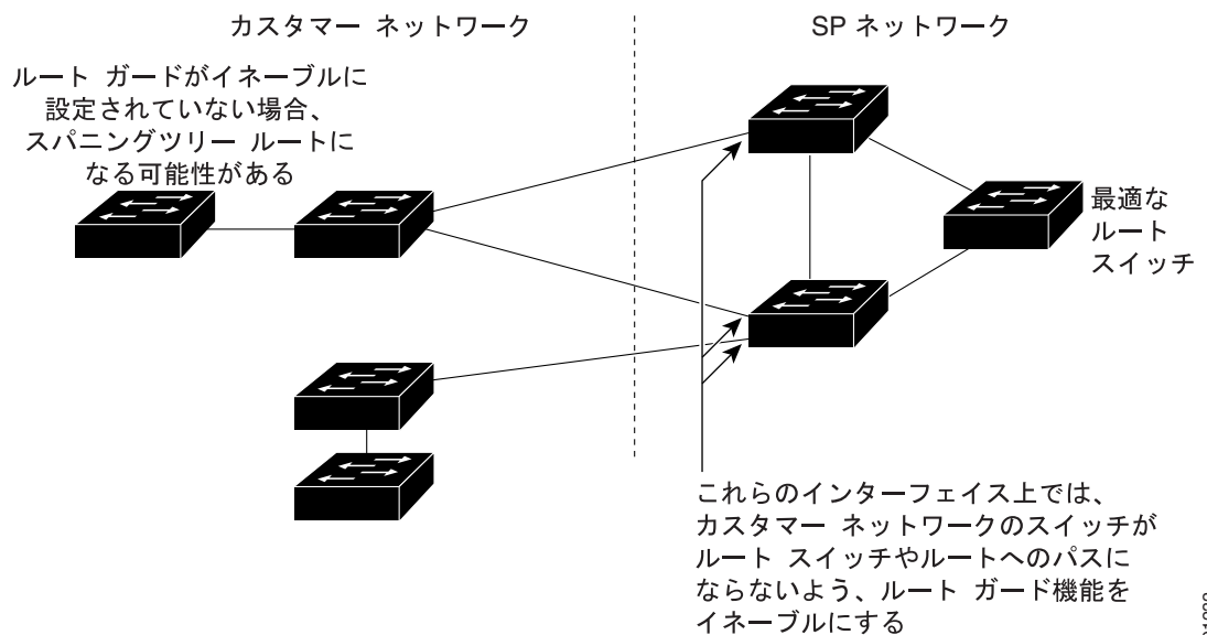
図 17-8 サービス プロバイダー ネットワークのルート ガード
