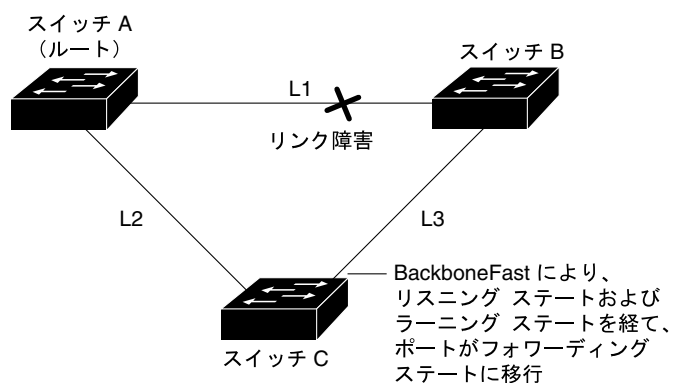
図 17-6 間接リンク障害発生後の BackboneFast の例
