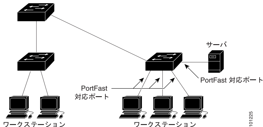
図 17-1 PortFast 対応インターフェイス
