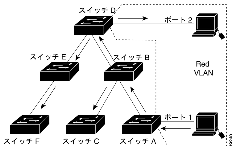
図 13-1 VTP プルーニングを使用しない場合のフラッディング ट्रフィック
