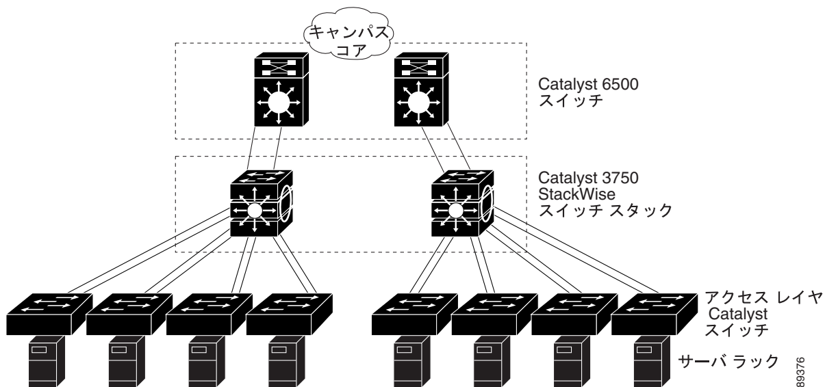
図 1-2 サーバ集約
