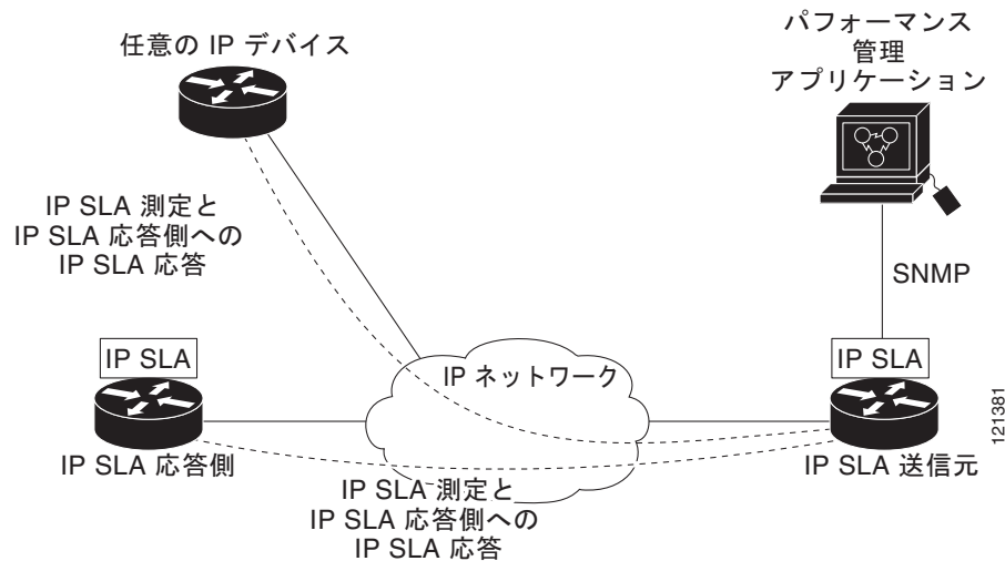
図 47-1 Cisco IOS IP SLA 動作
