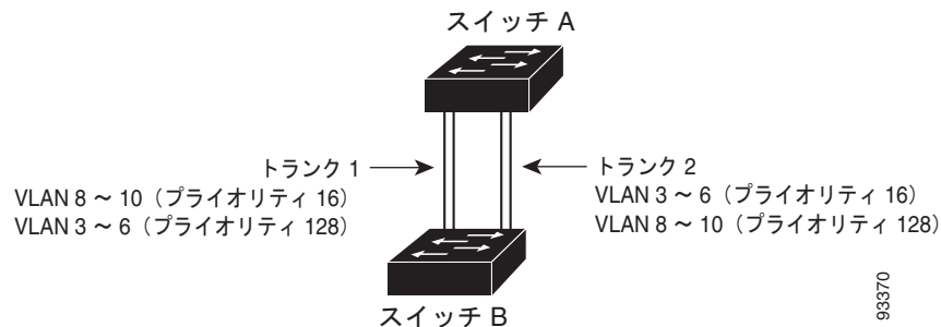
図 14-2 STP ポート プライオリティによる負荷分散
