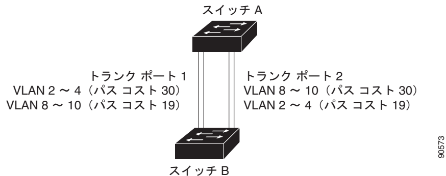
図 14-3 パス コストによってトラフィックが分散される負荷分散トランク
