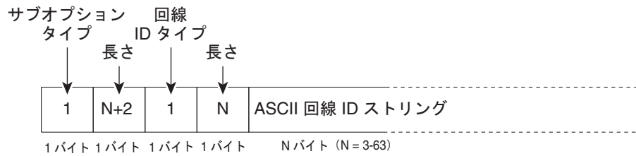
図 24-3 ユーザ設定のサブオプションのパケット形式
