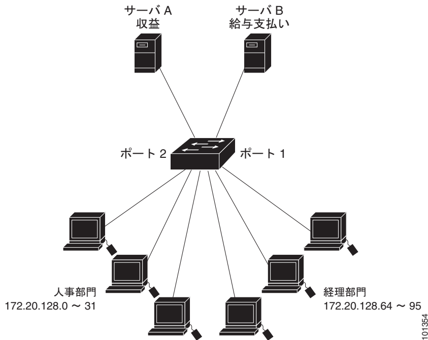
図 36-2 ルータ ACL によるトラフィックの制御
