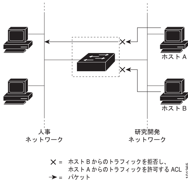
図 36-1 ACL によるネットワークへのトラフィックの制御
