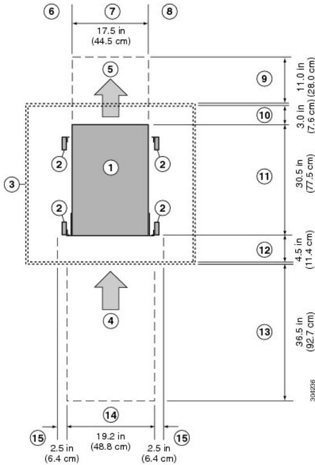
図 1: シャーシの周りに必要なスペース
