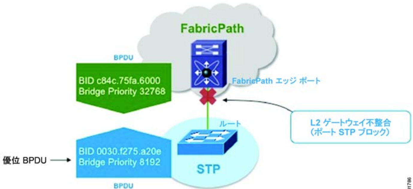
図 1-2 CE と FabricPath の例
