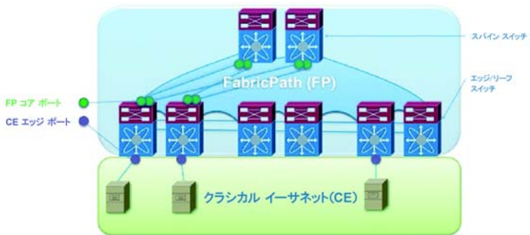
図 1-1 FabricPath トポロジの概要
