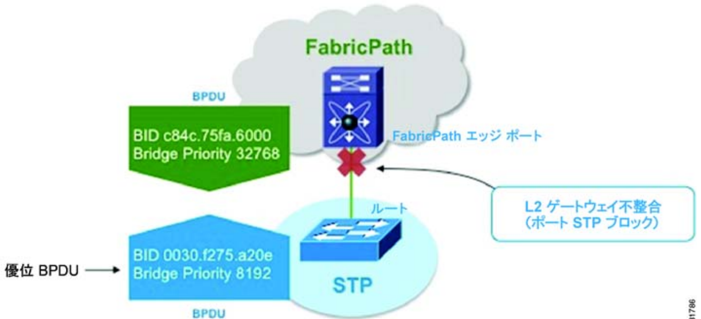
図 1-2 CE と FabricPath の例
