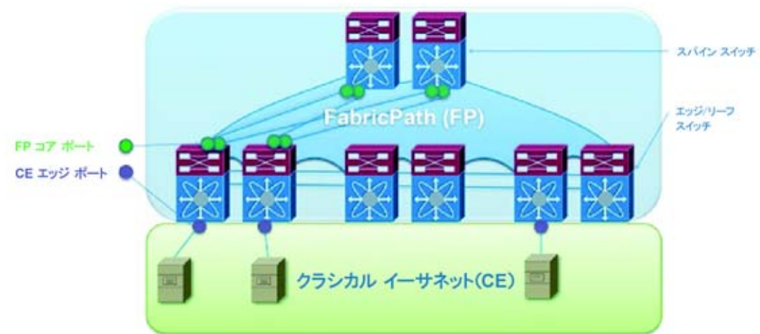
図 1-1 FabricPath トポロジの概要
