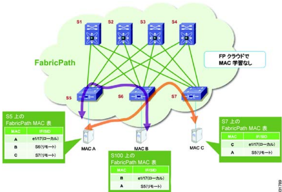
図 1-5 FabricPath を使用した MAC アドレス学習
