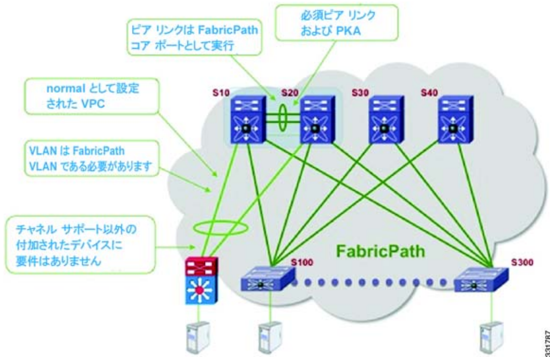
図 1-3 FabricPath の移行の例
