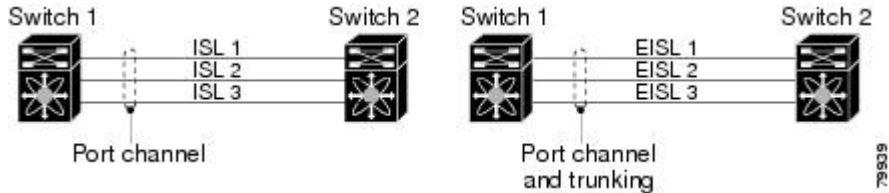
図 2: ポートチャンネルと VSAN トランキング
