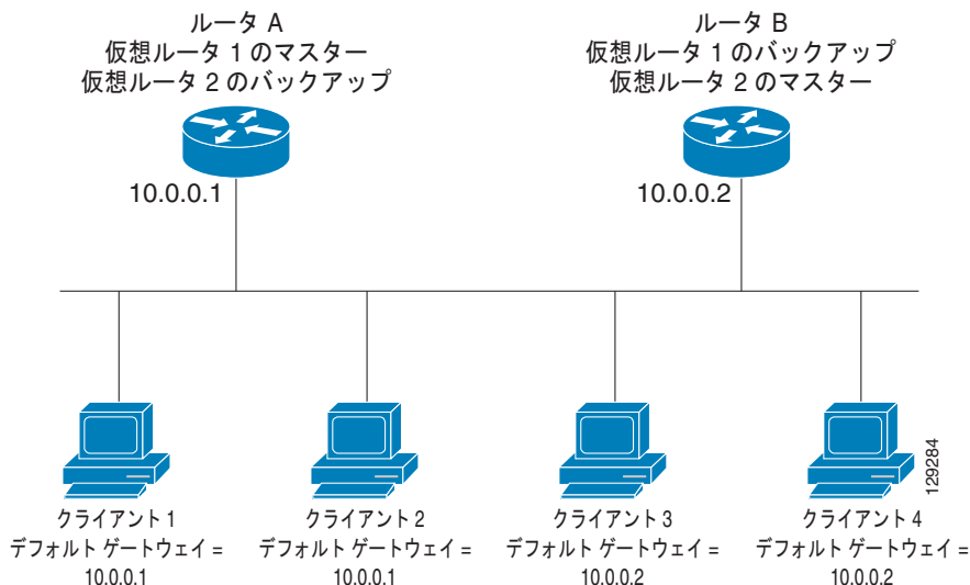
図 13-2 ロードシェアリングおよび冗長構成の VRRP トポロジ
