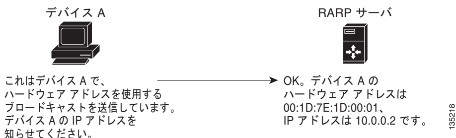
図 2-2 Reverse ARP
