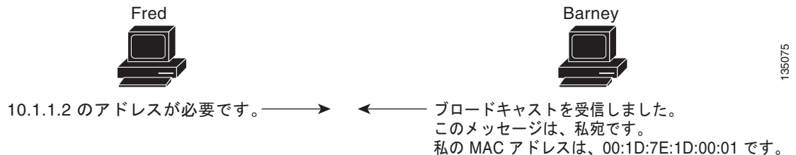
図 2-1 ARP 処理
