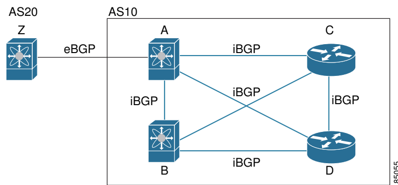
図 6-1 iBGP ネットワーク
