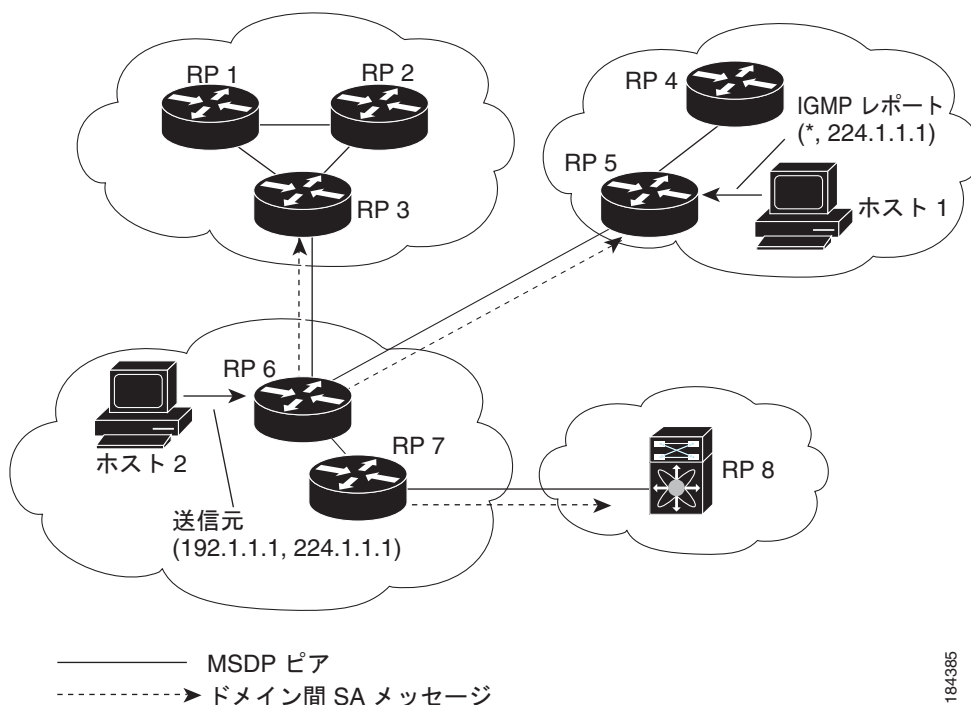
図 5-1 異なる PIM ドメインに属する RP 間の MSDP ピアリング
