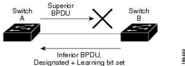
図 7: 単一方向リンク障害の検出
