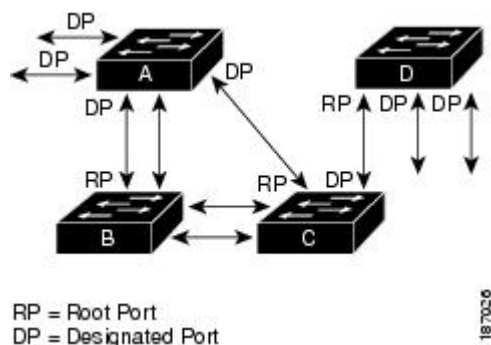
図 2: スパンニングツリートポロジ
