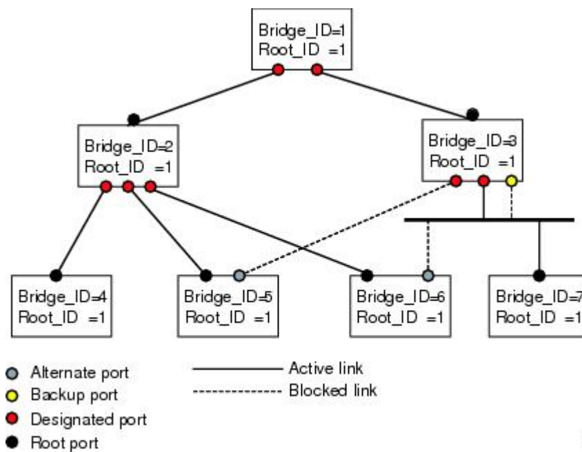
図 5：ポートのロールをデモンストレーションするトポロジのサンプル
