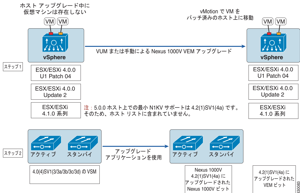
図 22 4.0(4)SV1(3、3a、3b、3c、3d) から 4.2(1)SV1(4a) へのアップグレード
