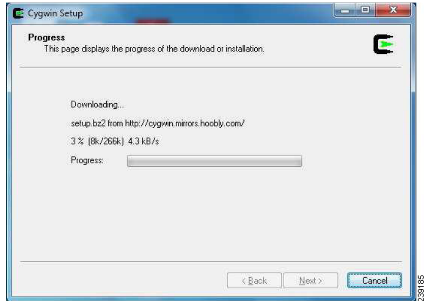
図 7 [Progress] 画面
