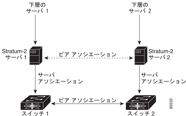
図 8-1 NTP のピアおよびサーバ アソシエーション
