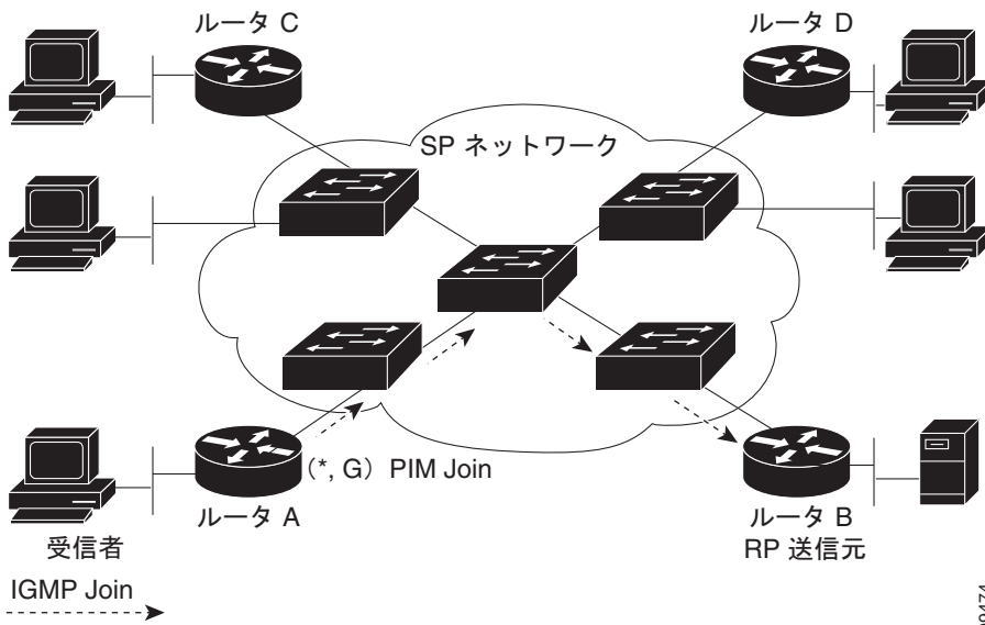
図 45-2 PIM スヌーピングがある場合の PIM Join メッセージフロー
