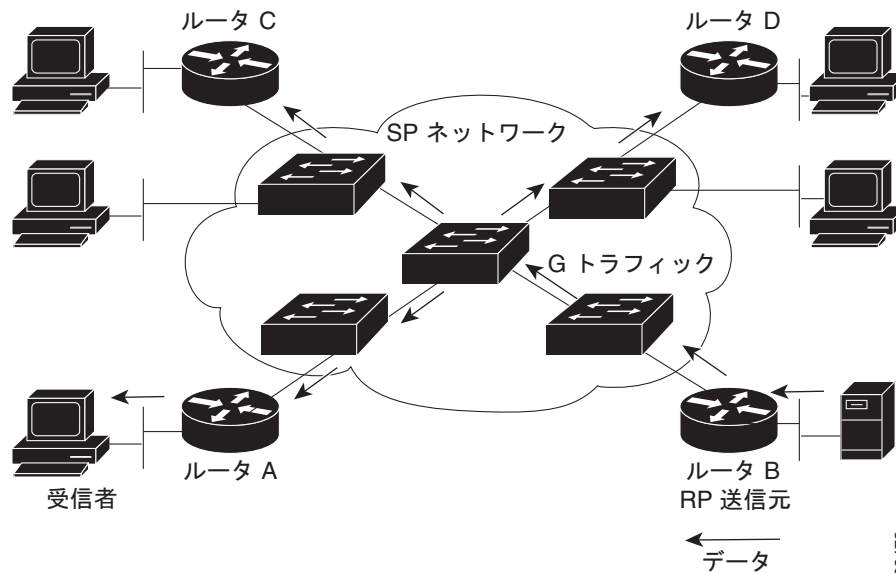
図 45-3 PIM スヌーピングがない場合のデータ トラフィック フロー
