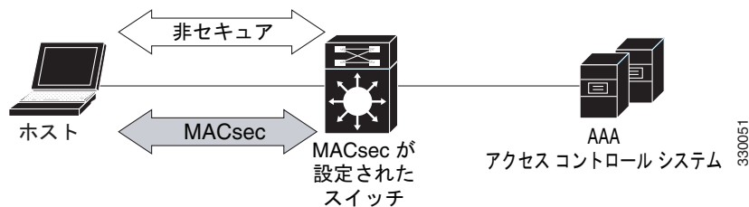
図 44-1 セキュアなデータ セッションでのシングルホスト モードの MACsec
