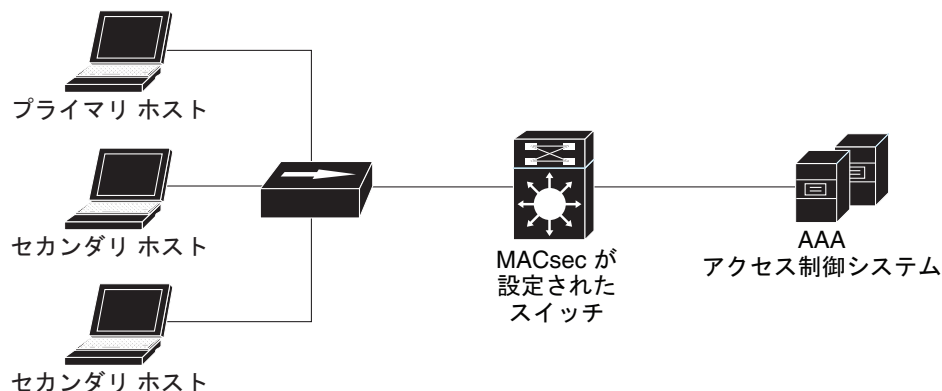
図 44-2 標準マルチホスト モードの MACsec : 非セキュア
